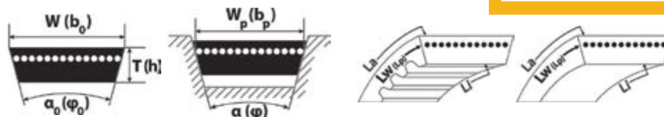
ГОСТ 24848.1-81 РЕМНИ КЛИНОВЫЕ ВАРИАТОРНЫЕ ДЛЯ ПРОМЫШЛЕННОГО ОБОРУДОВАНИЯ
