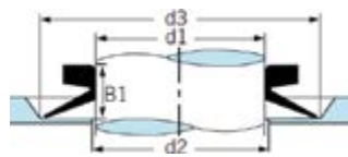
КОЛЬЦА V-RING ПРОФИЛЬ E
