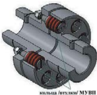
кольца /втулки/ МУВП
